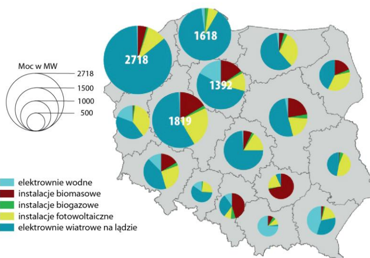
Rysunek 29. Moc elektryczna instalacji OZE powyżej 50 kW według województw z podziałem na technologie w MW, stan na 31 grudnia 2022 r.
