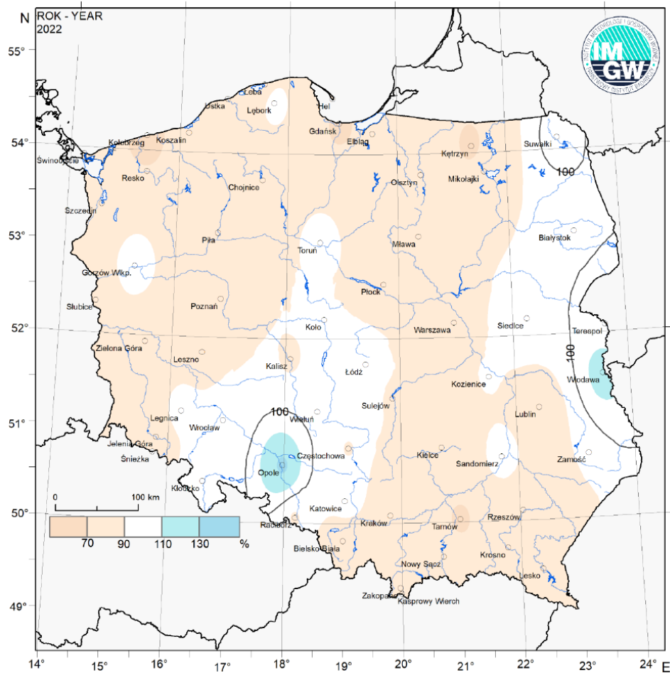
Rysunek 22. Anomalie rocznych sum opadów atmosferycznych w 2022 r. względem okresu referencyjnego 1991-2020
