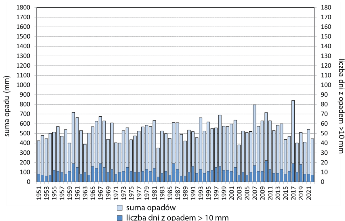
Rysunek 23. Zmienność wieloletnia rocznych sum opadów atmosferycznych oraz liczby dni z opadem >10 mm w roku na stacji synoptycznej w Szczecinie
